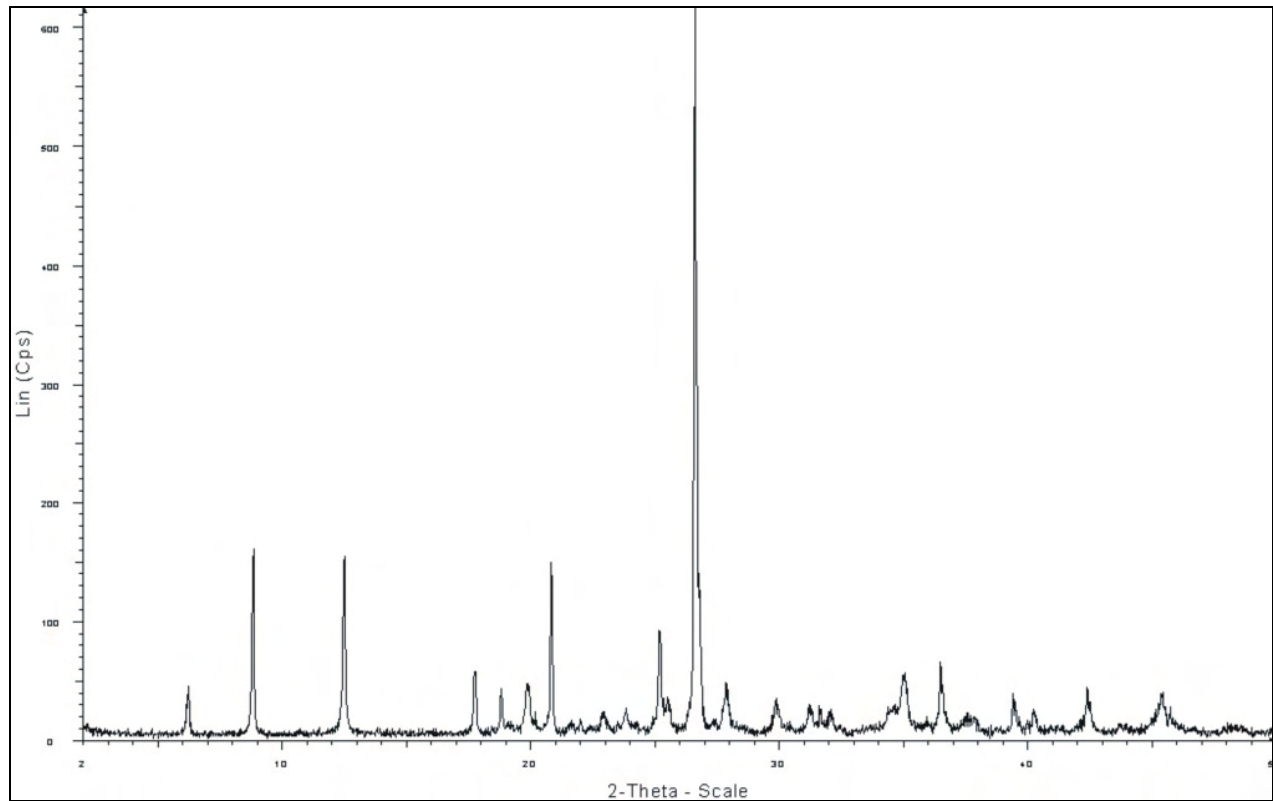
Diagramm 2: Pulveraufnahme
